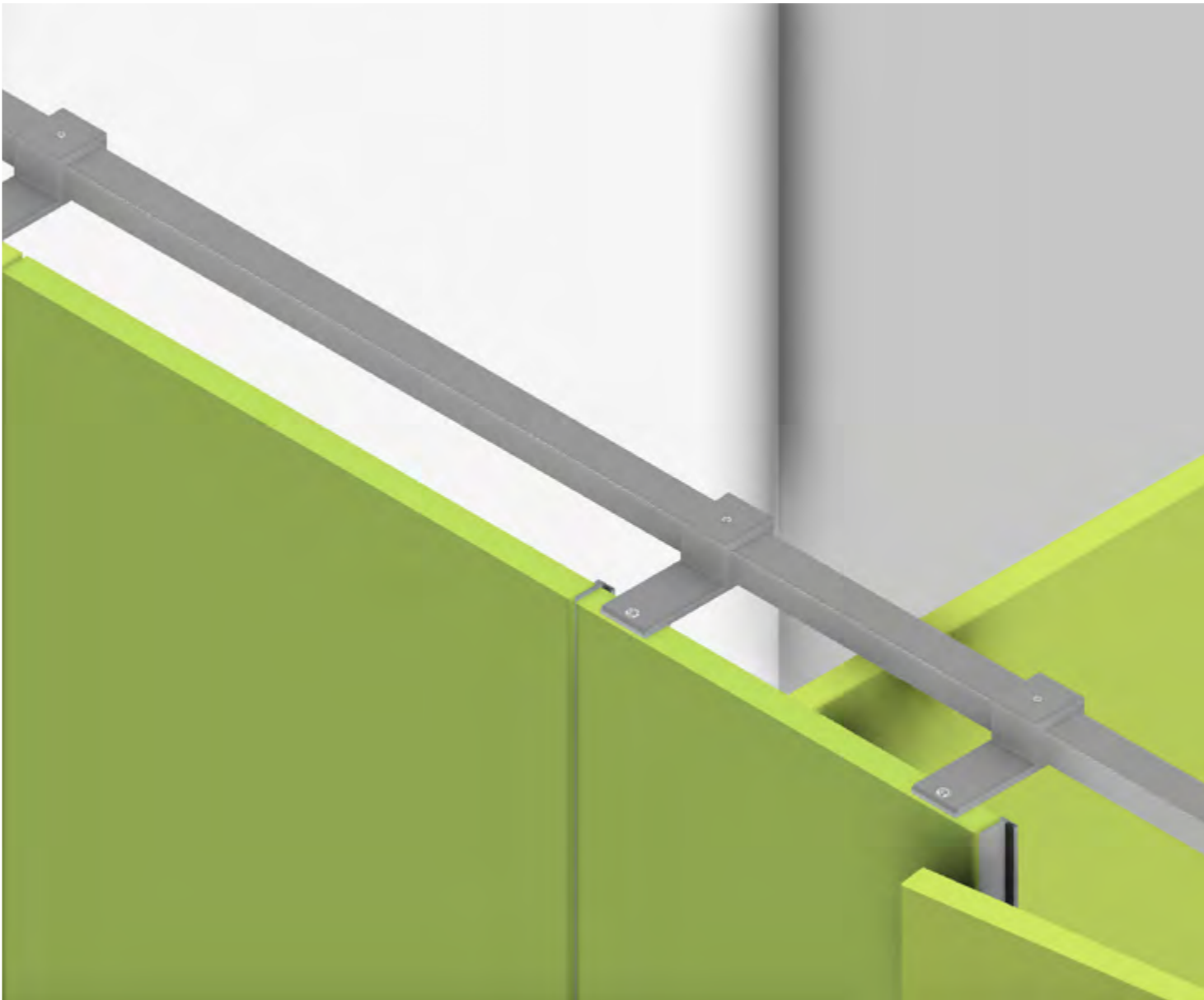
NiUU® one K schwebend mit zurückgesetztem Stabilisator, in Verkehrsweiß 9317
